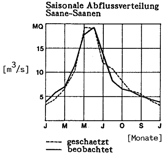
Fig. 4 Vergleich zwischen den geschätzten und den tatsächlich beobachteten langjährigen Monatsmitteln des Abflusses der Saane in Saanen
