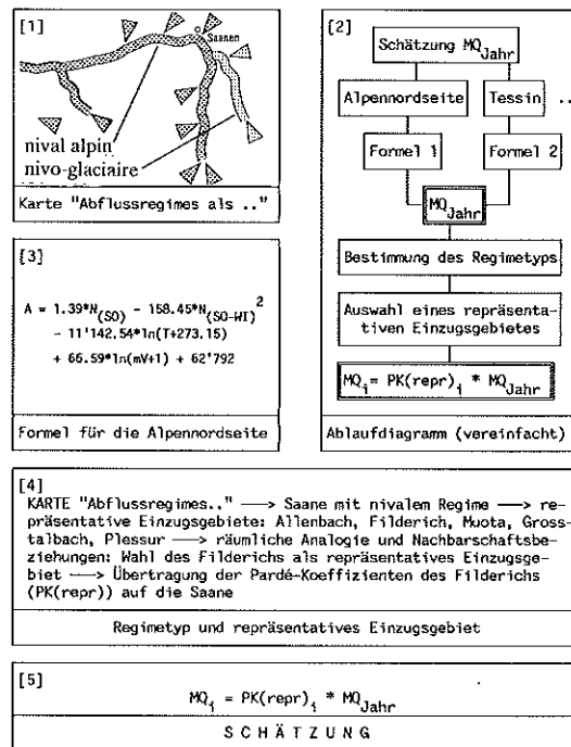
Fig. 3 Zur Abschätzung von langjährigen mittleren Monatsabflüssen mit Hilfe der Tafel «Abflussregimes» des «Hydrologischen Atlas der Schweiz» – Beispiel: Saane in Saanen; Abkürzungen: N SO : Gebietsniederschlag im Sommerhalbjahr [mm]; N SO-WI : Verhältnis Sommer- zu Wintergebietsniederschlag; T: mittlere Jahrestemperatur [°C]; mV: mittlere areale Vergletscherung [%]
