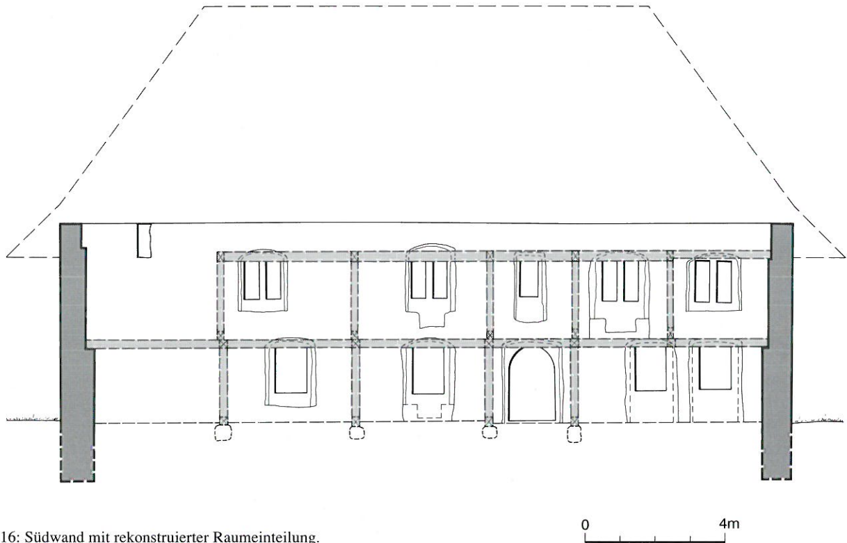
Abb. 16: Südwand mit rekonstruierter Raumeinteilung.
