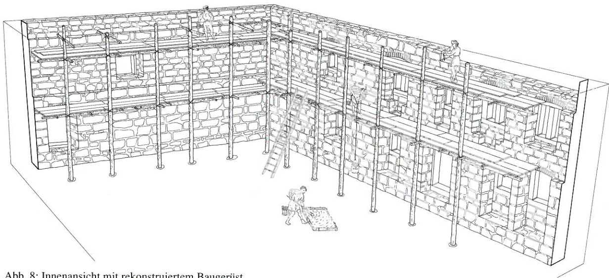
Abb. 8: Innenansicht mit rekonstruiertem Baugerüst.
