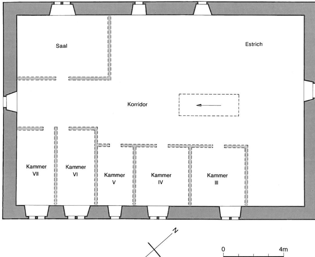
Abb. 42: Obergeschoss mit rekonstruierter Raumeinteilung.
