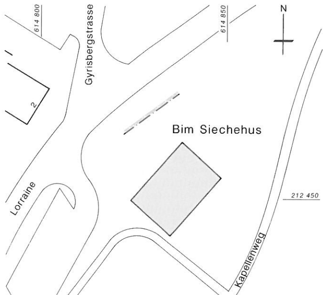
Abb. 47: Kanalisationssanierung, Situationsplan.
