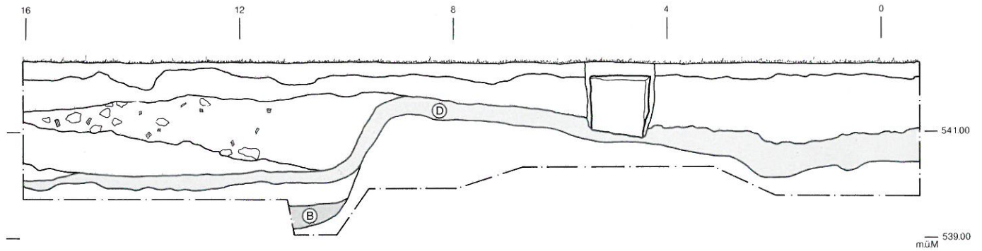
Abb. 48: Kanalisationssanierung, Südprofil.
