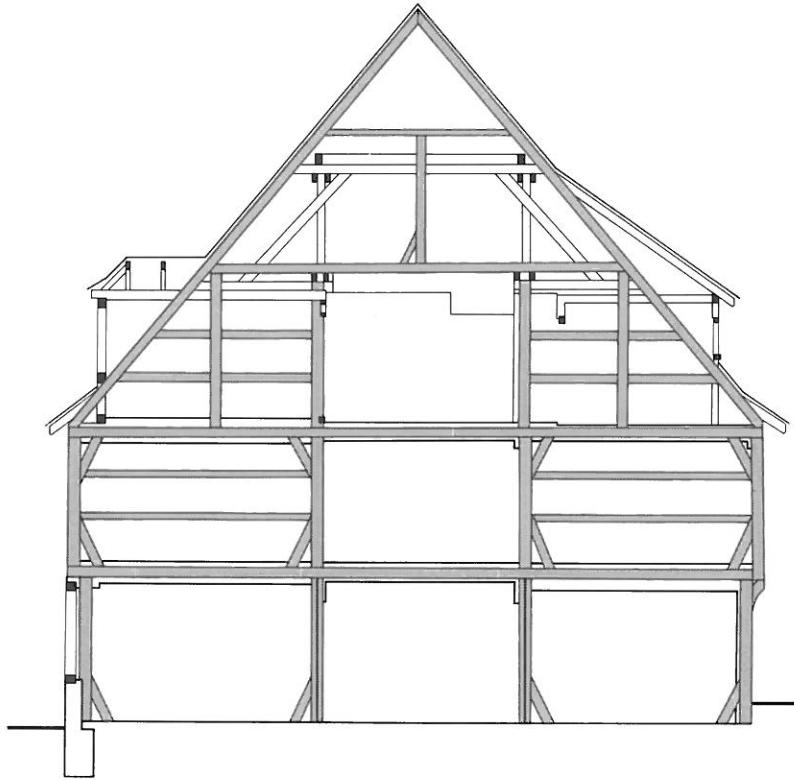
Abb. 50: Querschnitt des Siechenhauses in Steig mit rekonstruierter Raumaufteilung.
