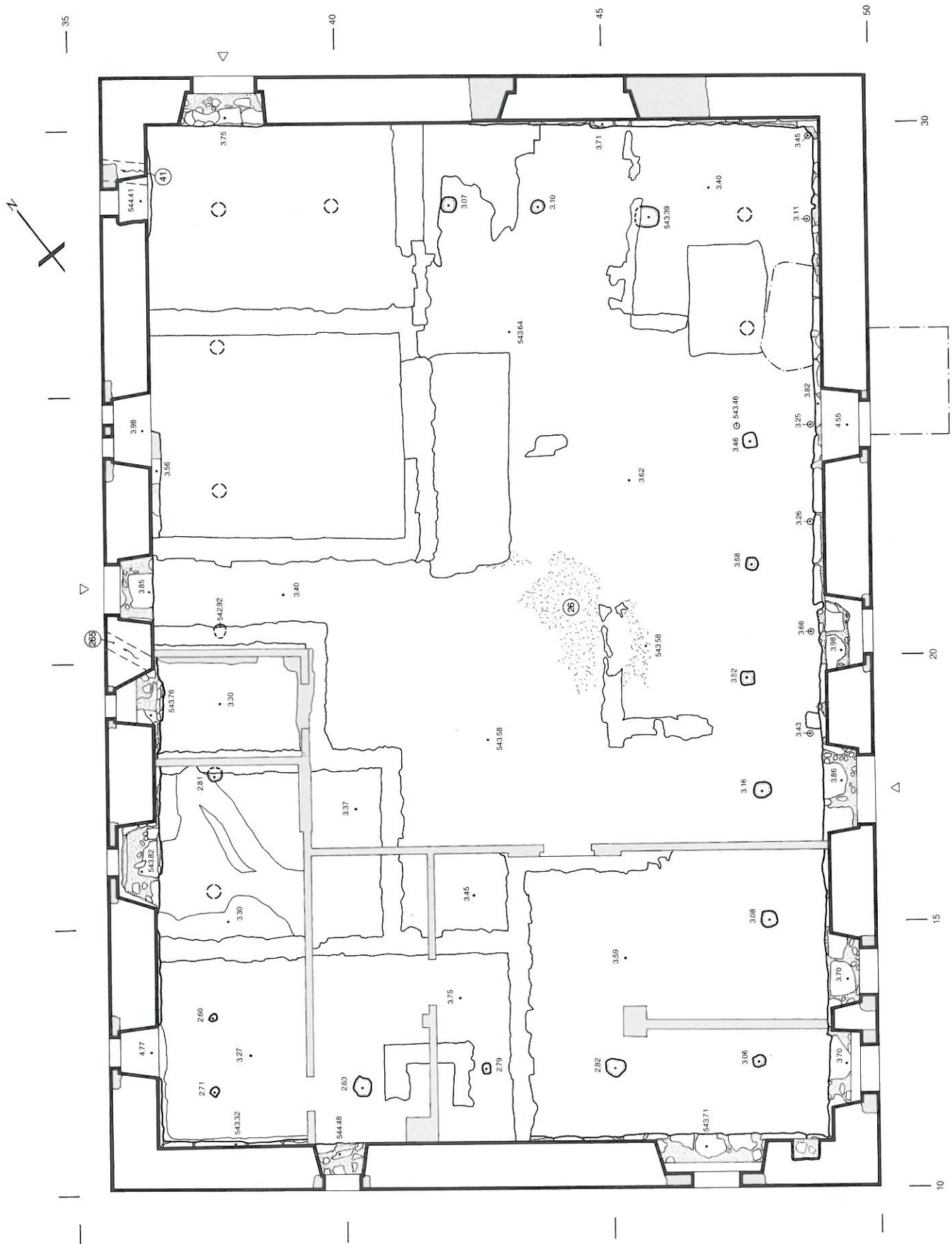
Tafel 6: Grundriss Erdgeschoss, Rohbau. M.1:100.
