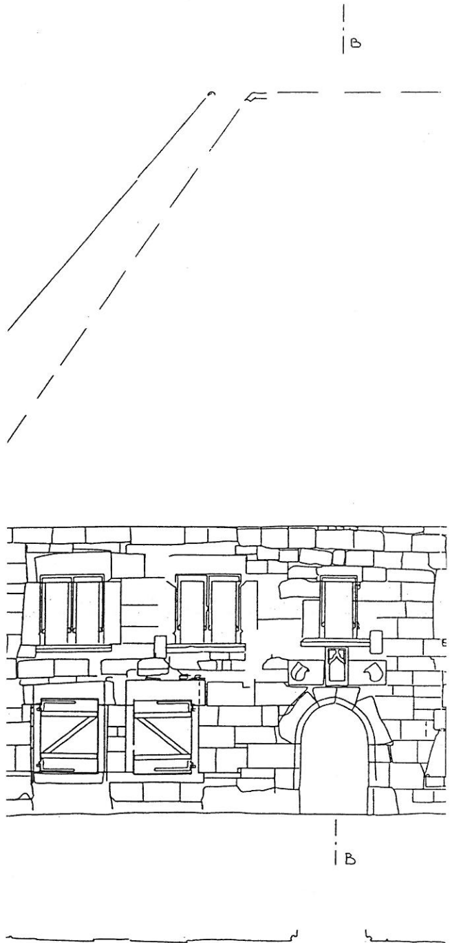
Abb. 4: Ausschnitt aus Südfassade (1:100). Büro de Waal, Hattem (NL).
