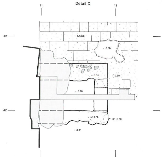
Abb. 25: Detail Feuerstelle, Phase 1.
