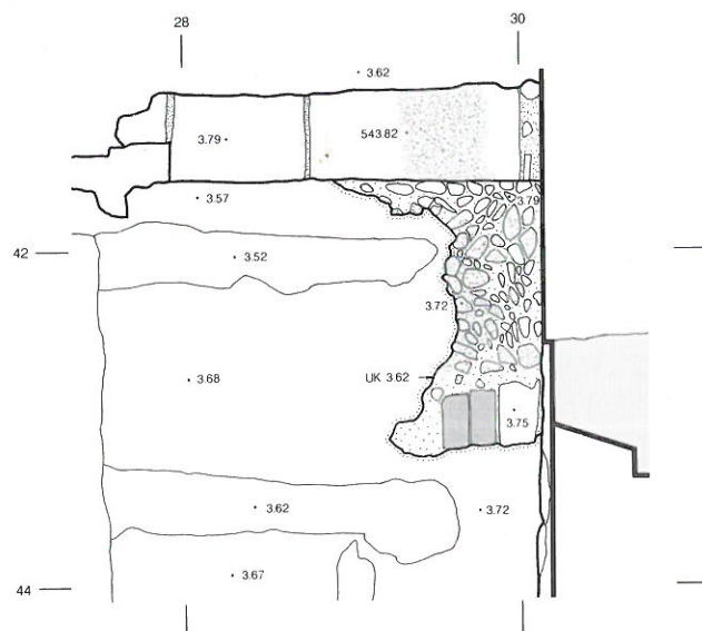
Abb. 36: Detail, Ofenanlage für Sudatio, jüngere Phase.
