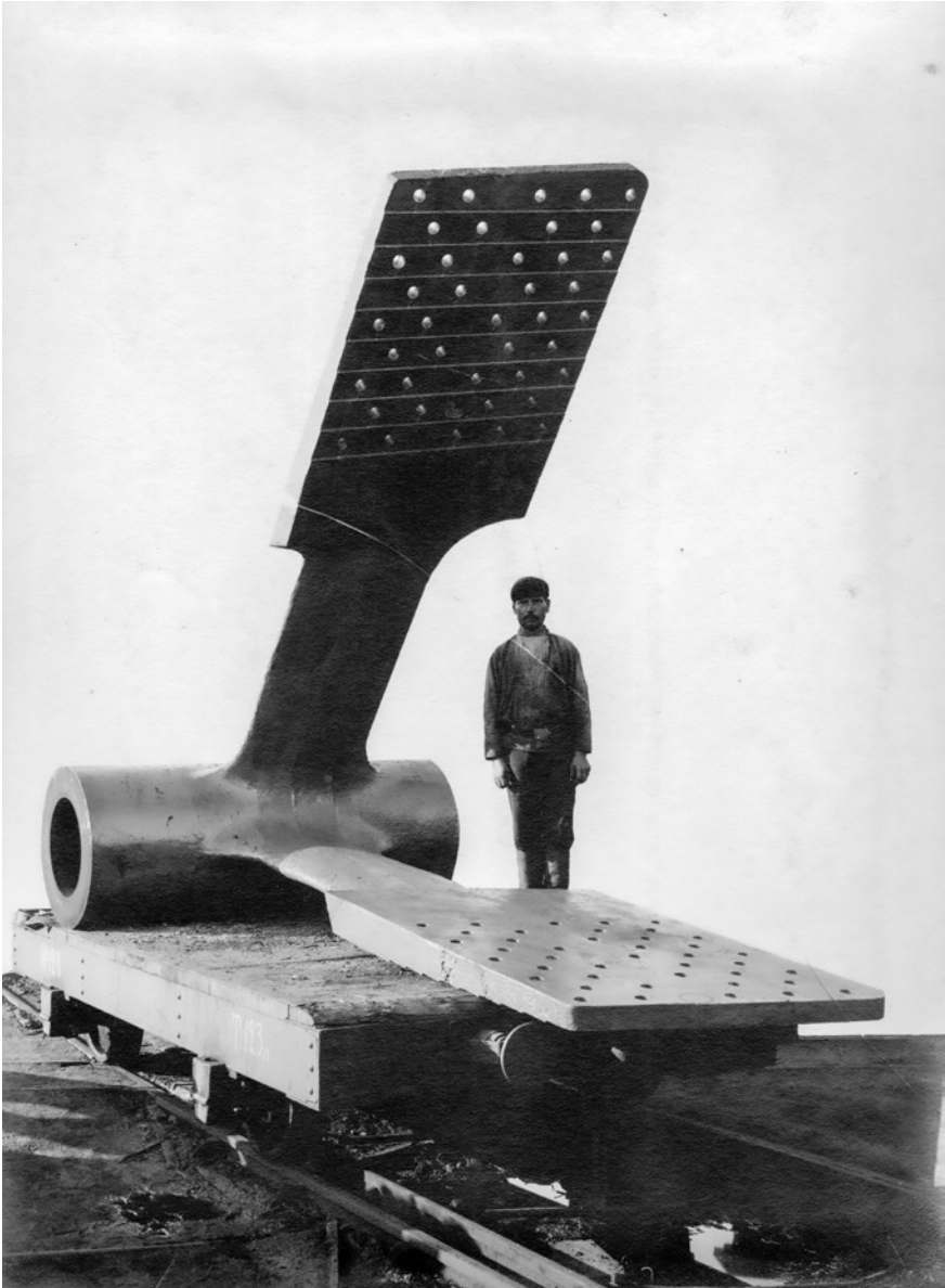
Abb. 24 o. A.: Großer Träger (Bol'soj kronštejn), in: o. A.: Kolomnaer Maschinenfabrik (Kolomenskij mašinostroitel'nyj zavod), o. O. 1916, S. 26. RNB OÉ È((ALTch100)/(2-2))
