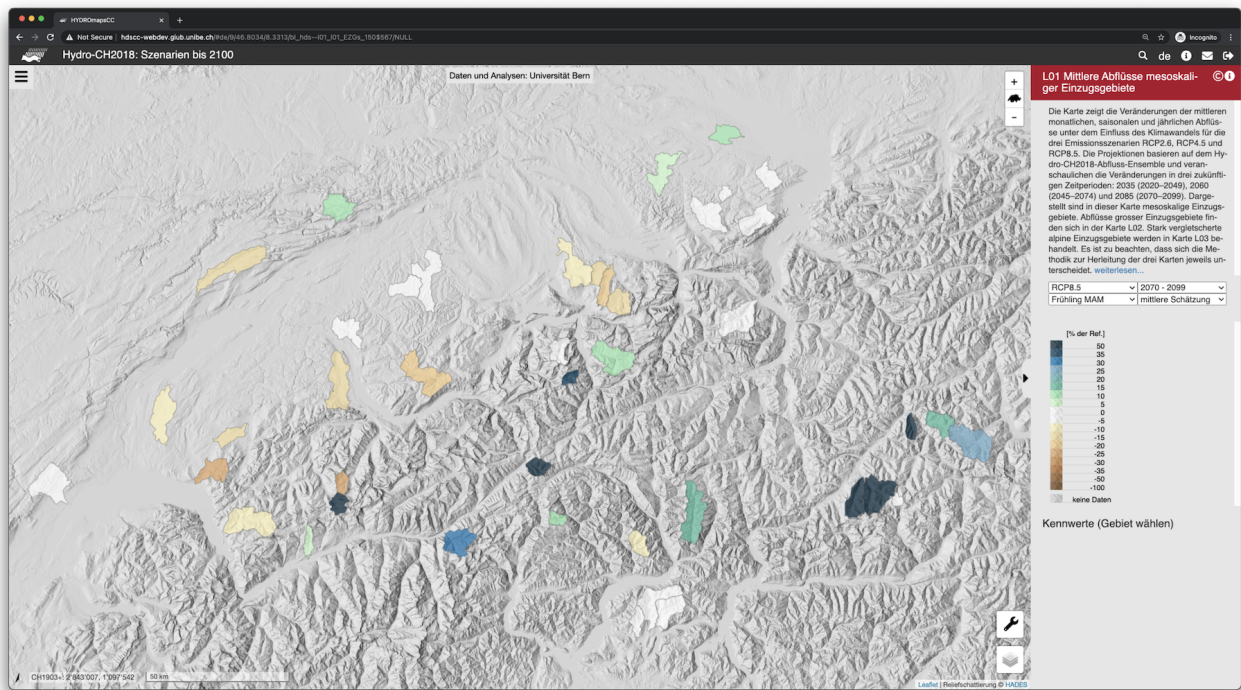
Abbildung 3. Relative Veränderungen der Frühlingsabflüsse bis Ende des 21. Jahrhunderts unter RCP8.5
