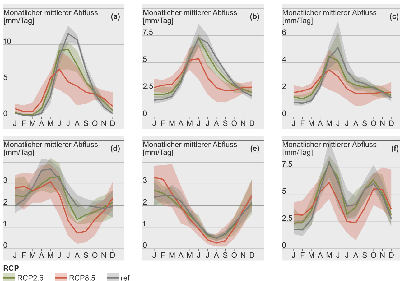
Abbildung 1. Die Abflussregimes von Rosegbach (a), Kander (b), Plessur (c), Emme (d), Venoge (e) und Verzasca (f). Die dick ausgezogenen Linien zeigen den Mittelwert aller Modelle für die Referenzperiode (grau), für 2085 unter RCP2.6 (grün) und für 2085 unter RCP8.5 (rot). Der schattierte Bereich zeigt die gesamte Bandbreite aller Modelle [11].
