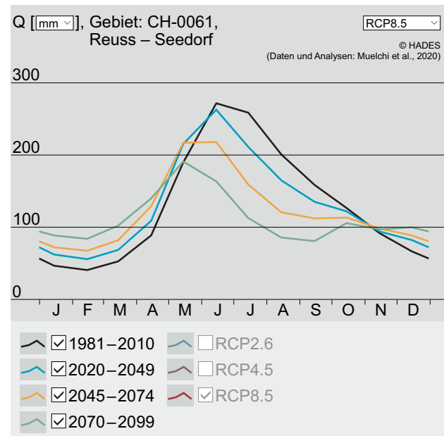
Abbildung 2. Reuss–Seedorf: Veränderung des Abflussregimes bis Ende des 21. Jahrhunderts
