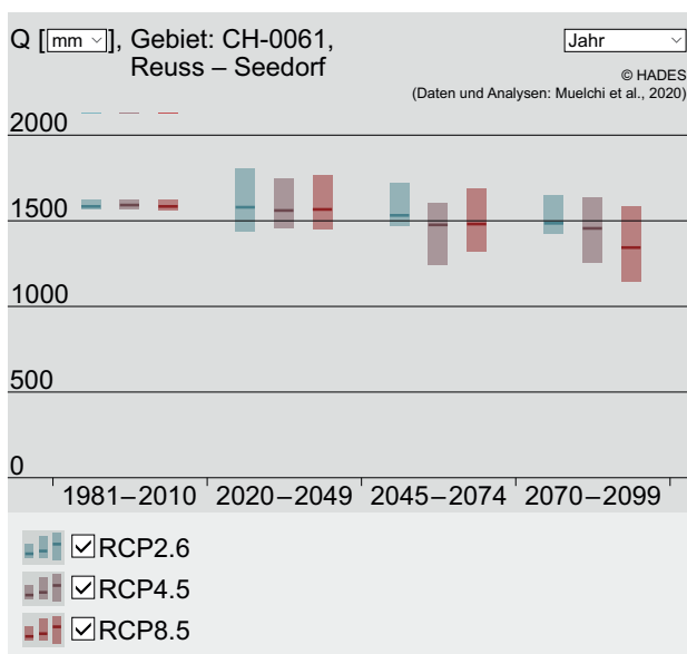
Abbildung 4. Reuss–Seedorf: Abnahme des Jahresabflusses bis Ende des 21. Jahrhunderts unter RCP2.6 (blau), RCP4.5 (violett) und RCP8.5 (rot)
