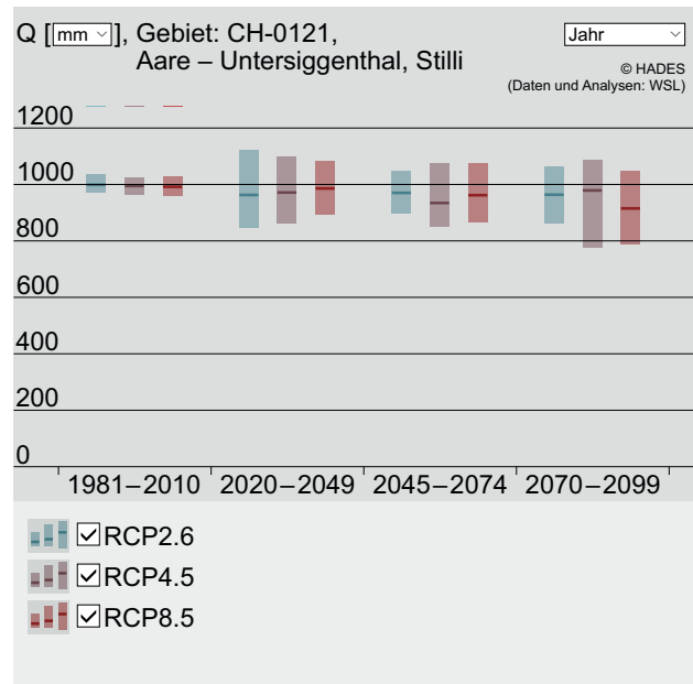
Abbildung 2. Aare–Untersiggenthal, Stilli: Abnahme der Jahresabflüsse bis Ende des 21. Jahrhunderts, unterteilt nach den drei Emissionsszenarien RCP2.6, RCP4.5 und RCP8.5
