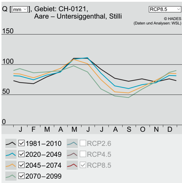
Abbildung 1. Aare–Untersiggenthal, Stilli: Veränderung des Abflussregimes bis zum Ende des 21. Jahrhunderts unter dem Emissionsszenario RCP8.5, beginnend in schwarz (Referenzperiode) über blau (2035) und gelb (2060) und endend in grün (2085)
