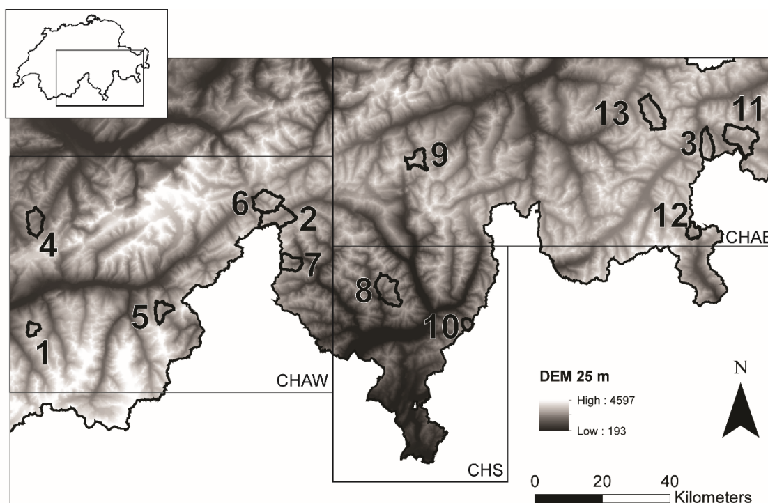
Figure 2 : Emplacements des bassins versants utilisés dans cette étude. Le bassin de recherche du CHYN/Crealp (Vallon de Rechy) correspond au No. 1 (Arnoux et al. 2020a).
