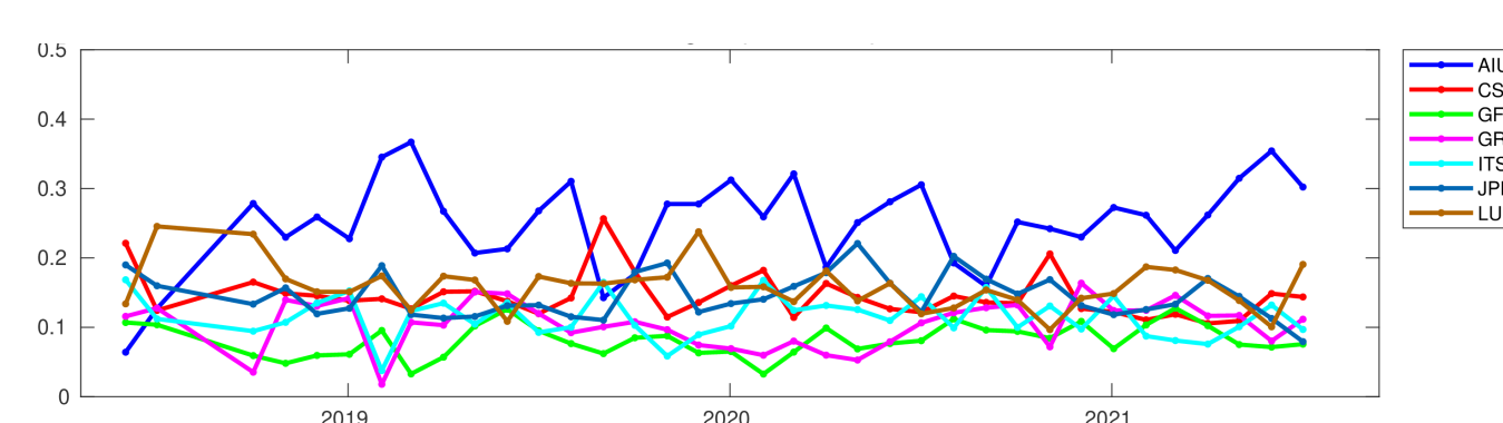
Abbildung 6: Gewichte, mit denen verschiedene monatliche GRACE-FO Lösungen in eine kombinierte Lösung einfließen. Die Kombination wird im Rahmen von COST-G am AIUB operationell gemacht. Für die meisten Monate trägt die am AIUB gerechnete Einzellösung am stärksten bei.
