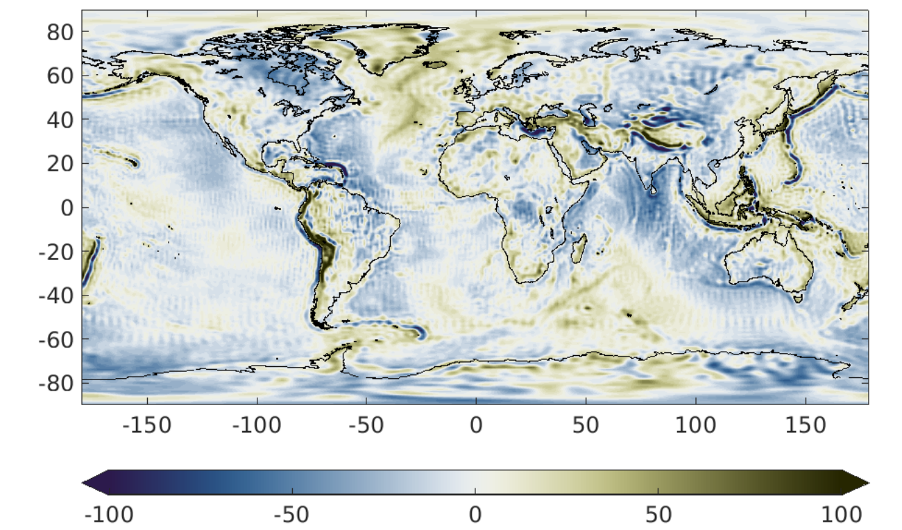
Abbildung 8: Abweichungen der lokalen Schwerebeschleunigung von einer theoretischen Beschleunigung wenn die Erde ein Rotationsellipsoid wäre. Einheiten: mGal = 0.00001 m/s 2 .
