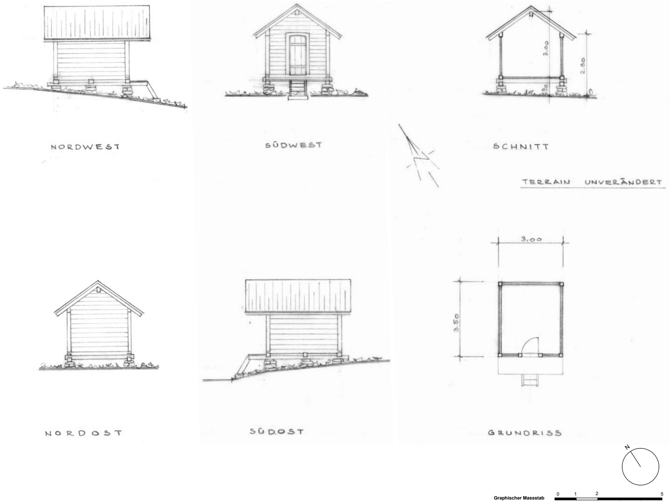
7 Freilichtmuseum der Schweiz, Kornspeicher aus Montsevelier: Plan für die Baueingabe zur Errichtung des Museumsgebäudes. Das grundlegende Konstruktionsprinzip des Kornspeichers lässt sich daran nachvollziehen. Ohne Datum.
