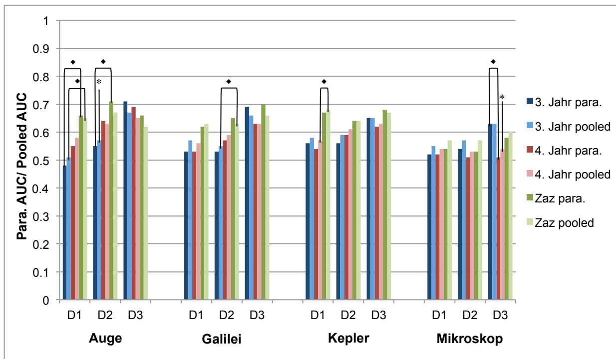
Abbildung 6: Graphische Darstellung der parametrischen (para.) und gepoolten (pooled) AUC-Werten der verschiedenen Untersucherguppen bei den unterschiedlichen Diagnostik-Schwellen ( D_1 - D_3 ) und verschiedenen Untersuchungshilfsmittel. Signifikante Unterschiede wurden mit einem ♦ markiert, während signifikante Unterschiede einer Gruppe zu den beiden anderen Gruppen mit einem * gekennzeichnet worden sind ( p < 0.05 ).
