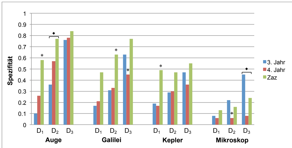
Abbildung 2: Spezifitäten der verschiedenen Untersucherguppen bei den unterschiedlichen Diagnostik-Schwellen ( D_1 - D_3 ). Die Resultate der Gruppen wurden jeweils zusammengefasst und als Mittelwerte (nach parametrischer Modellierung) dargestellt. Signifikante Unterschiede einer Gruppe zu den beiden anderen Gruppen wurden mit einem * gekennzeichnet, während signifikante Unterschiede zwischen allen Gruppen mit einem ♦ markiert sind ( p < 0.05 ).
