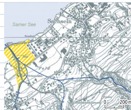
Fig. 12: Carte des dangers de Sachseln 2000 (© OFEG)
