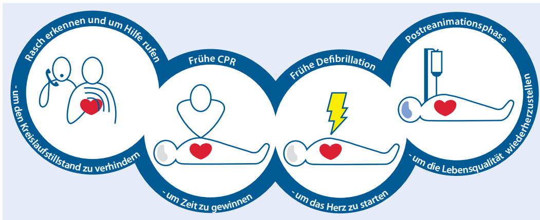
Abb. 2 ◀ Überlebenskette
