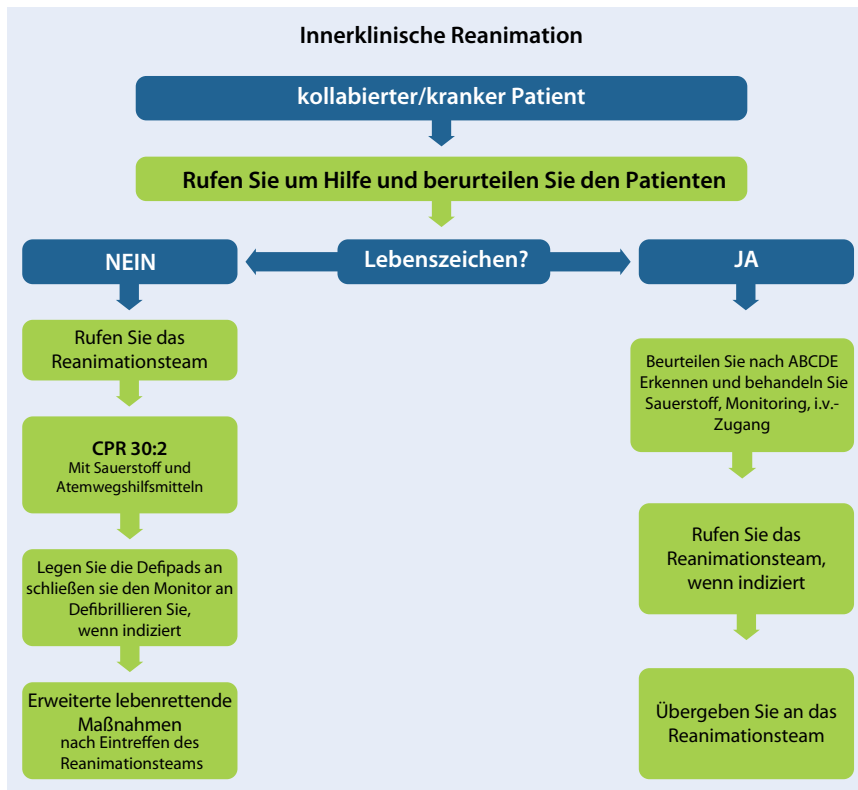
Abb. 6 ▲ „In-hospital resuscitation“
